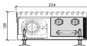
Modèle FAN 224 – 109
