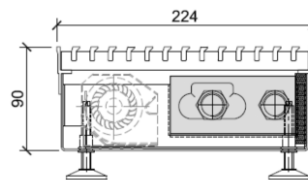
Modèle FAN 224-090
