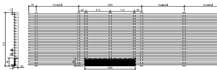
Grille linéaire 1610 - B (porte coulissant)
