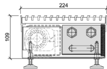
Modell FAN 224-109 (Anschluss seitlich)
