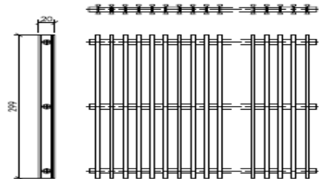
Rollrost Typ 941 – 17 -B
