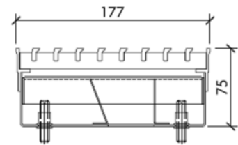
Modell SOL 177-075 (Anschluss von unten)
