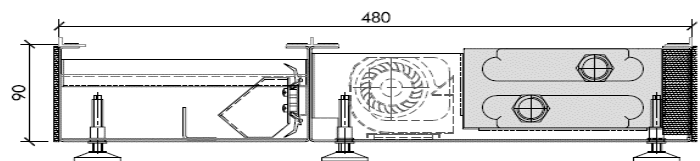
Modell FAN 480 – 90 (Anschluss seitlich)
