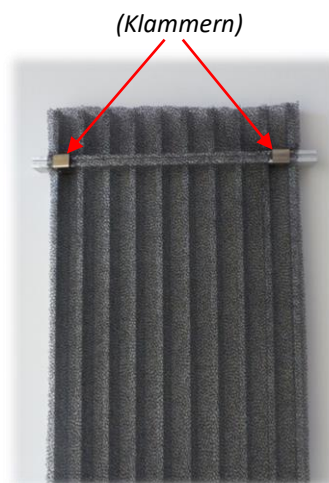
Bild 2 Gitter mit Filtervlies (Rückseite)
